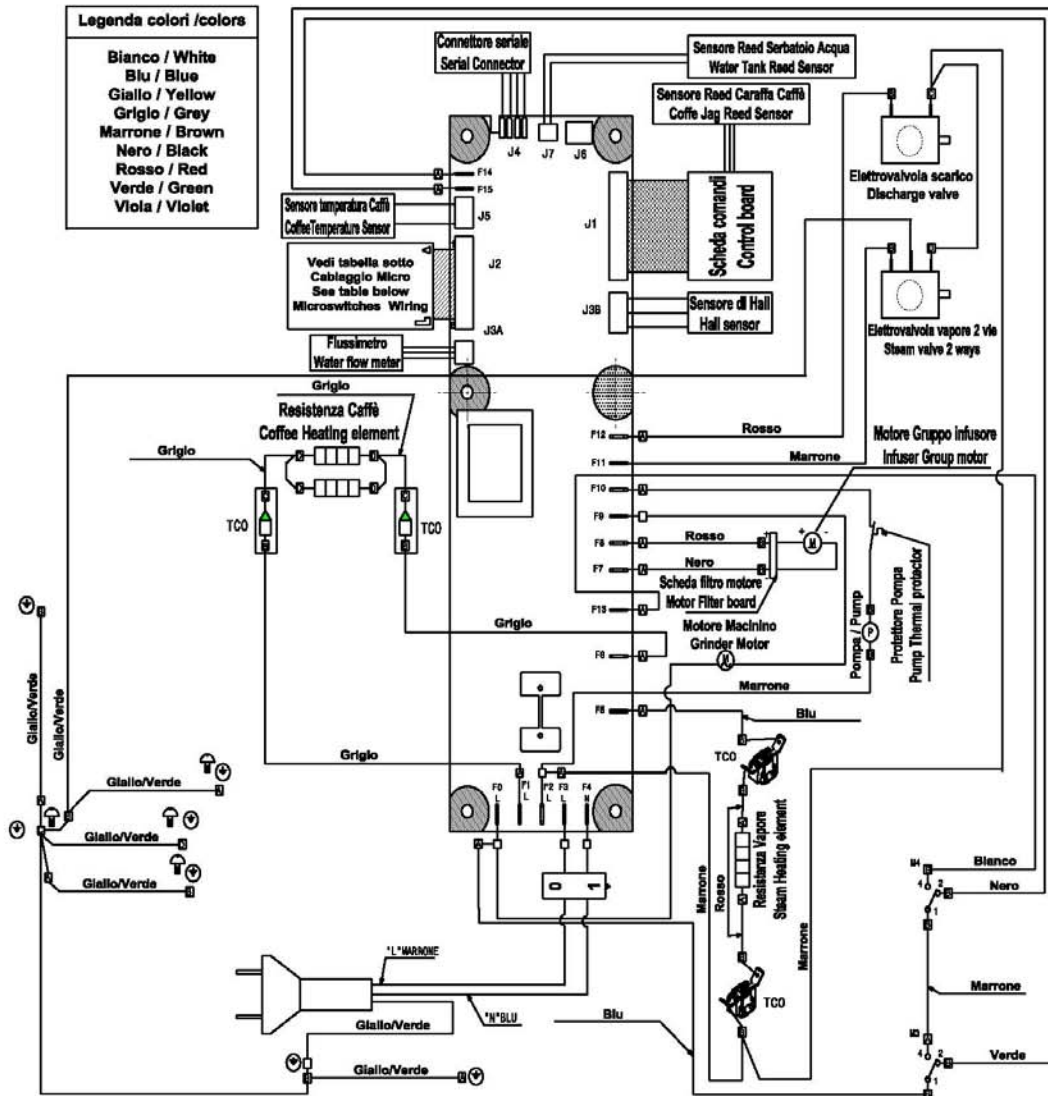
Cablaggio Micro / Microswitches Wiring
