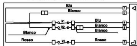
Cablaggio Micro / Microswitches Wiring
